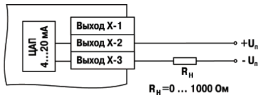
Рис. Б.5. Схема подключения нагрузки к ВУ типа И
