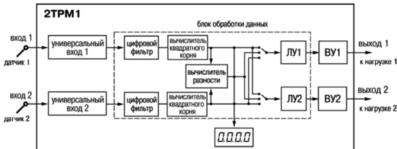
Рис. 3.1. Структурная схема прибора
