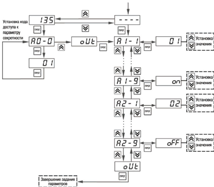
Рис. 6.3. Последовательность работы с прибором на втором уровне программирования (для группы параметров A)
