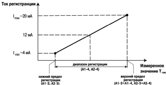
Рис. 3.14. Принцип формирования тока регистрации
