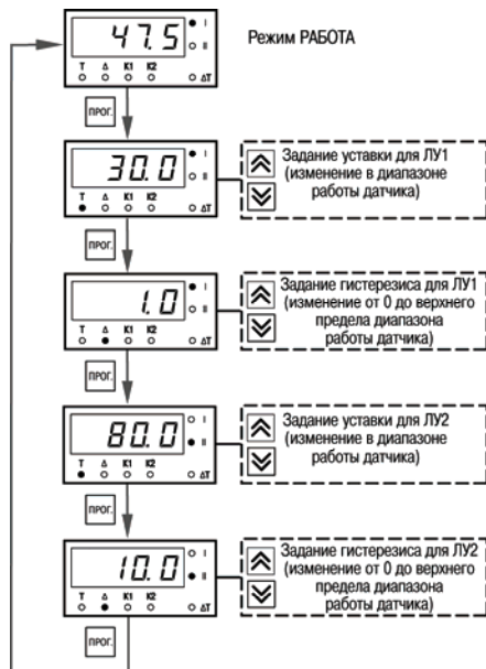
Рис. 6.1. Последовательность работы с прибором на первом уровне программирования
