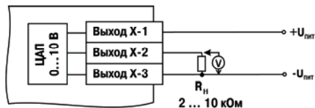
Рис. Б.6. Схема подключения нагрузки к ВУ типа У
