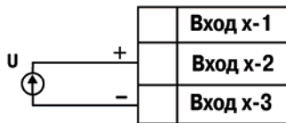
Рис. Б.10. Схема подключения активного датчика с выходом в виде напряжения -50 ... 50 мВ или 0 ... 1 В
