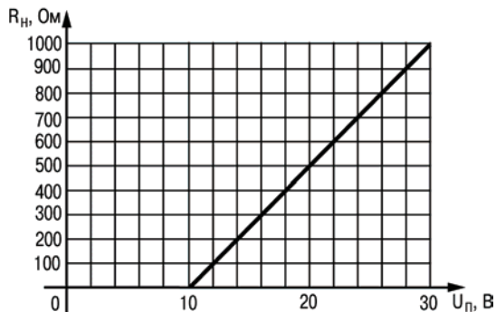
Рис 3.16. График зависимости R_n(U_n)
