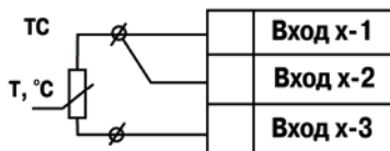
Рис. Б.8. Схема подключения термометра сопротивления
