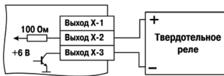
Рис. Б.7. Схема подключения к ВУ типа Т
